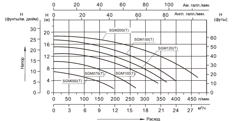
Кривые характеристик
