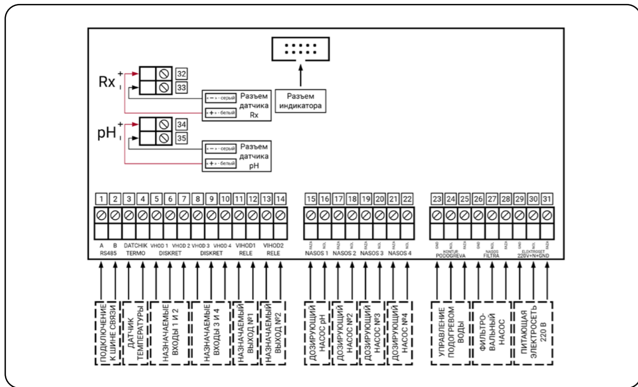
Рис.3 - Электрические подключения DOZBOX 2
